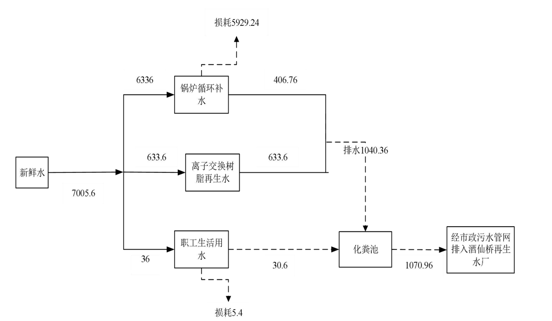
图8 本项目水平衡图（单位： m³/a）
