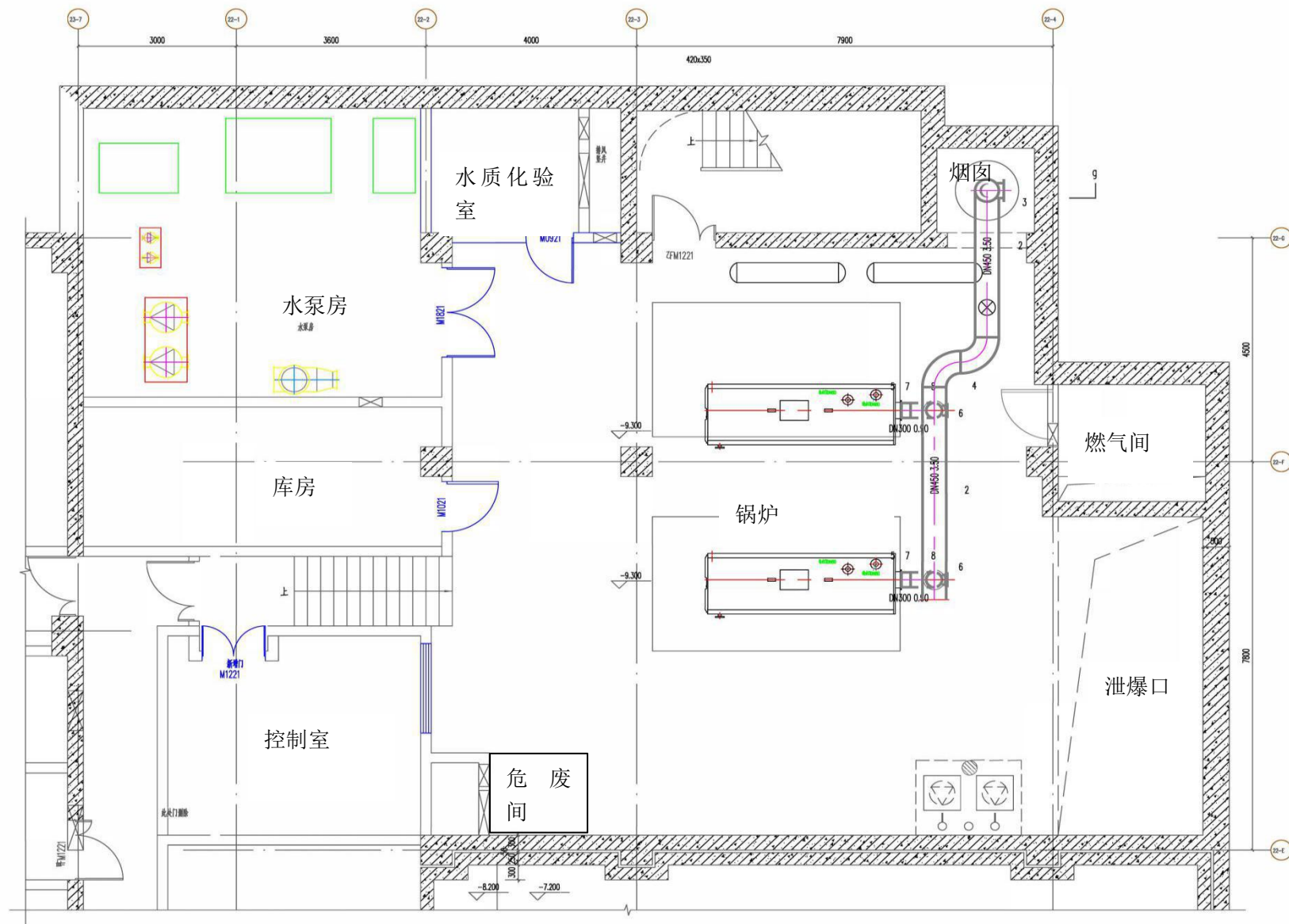
图4 锅炉房平面布置图 (1:50)
