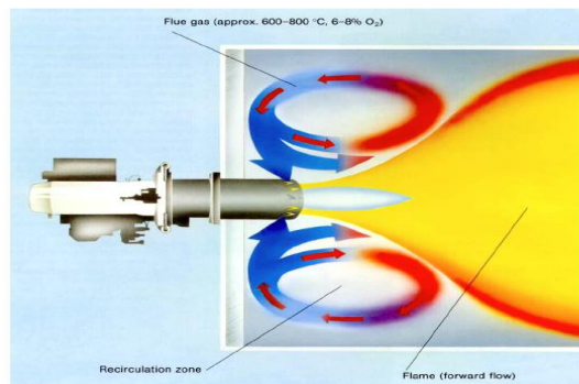
低氮氧燃烧器—炉膛内部火焰
