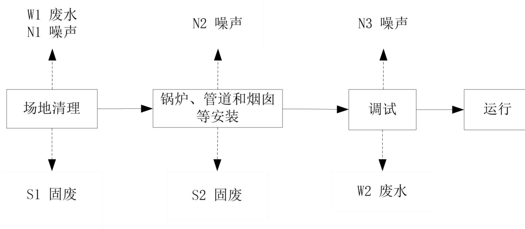
图6 施工期工艺流程及产污节点图
